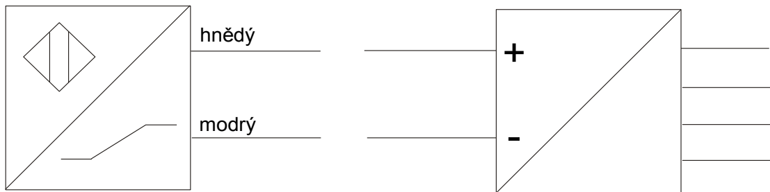
Obr.7: Příklad zapojení snímače NAMUR
