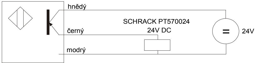
Obr.5: Příklad zapojení snímače s výstupem PNP trojdrát
