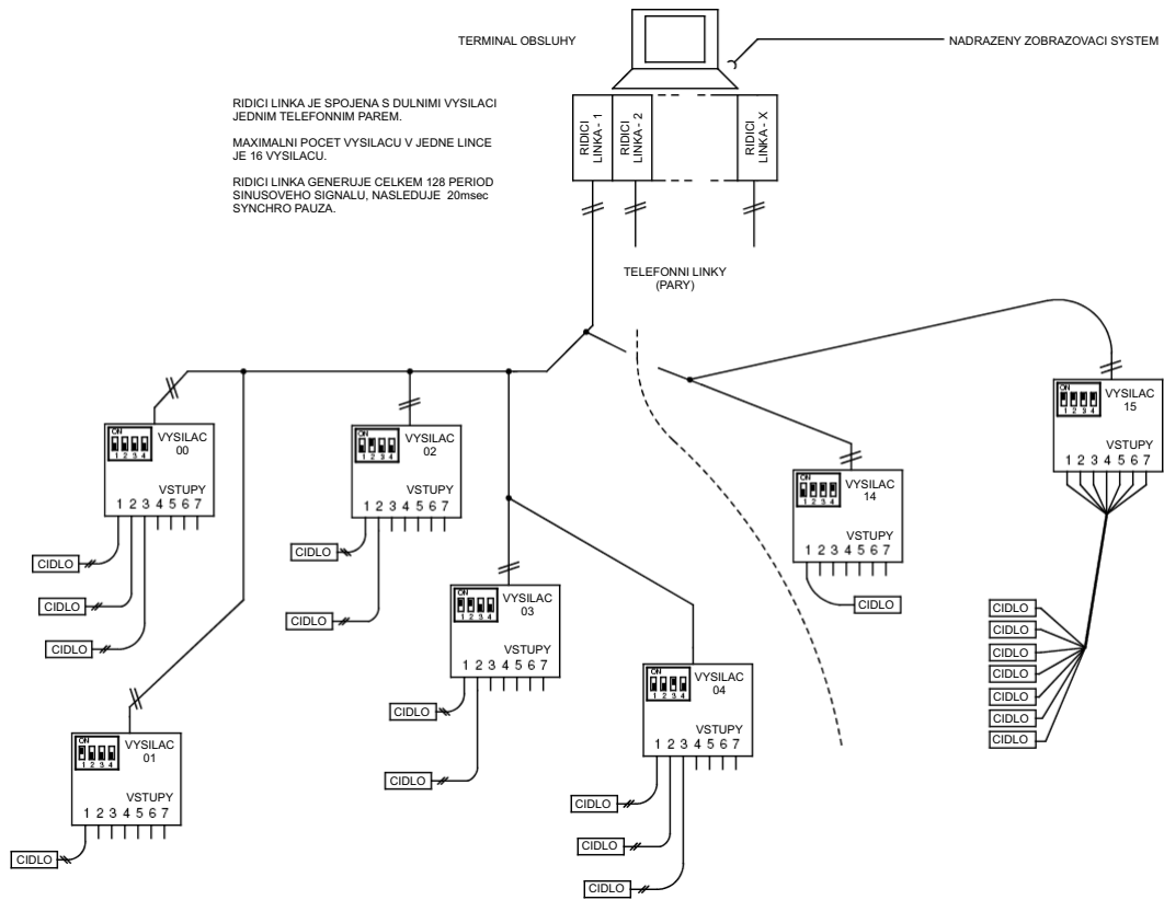
Blokové schéma systému
