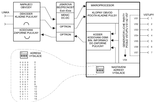
Blokové schéma vysílače
