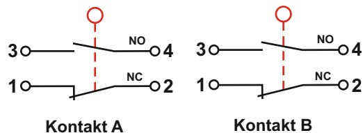
Kontakty spínače
