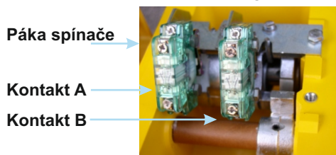
Řazení kontaktů ve spínači
